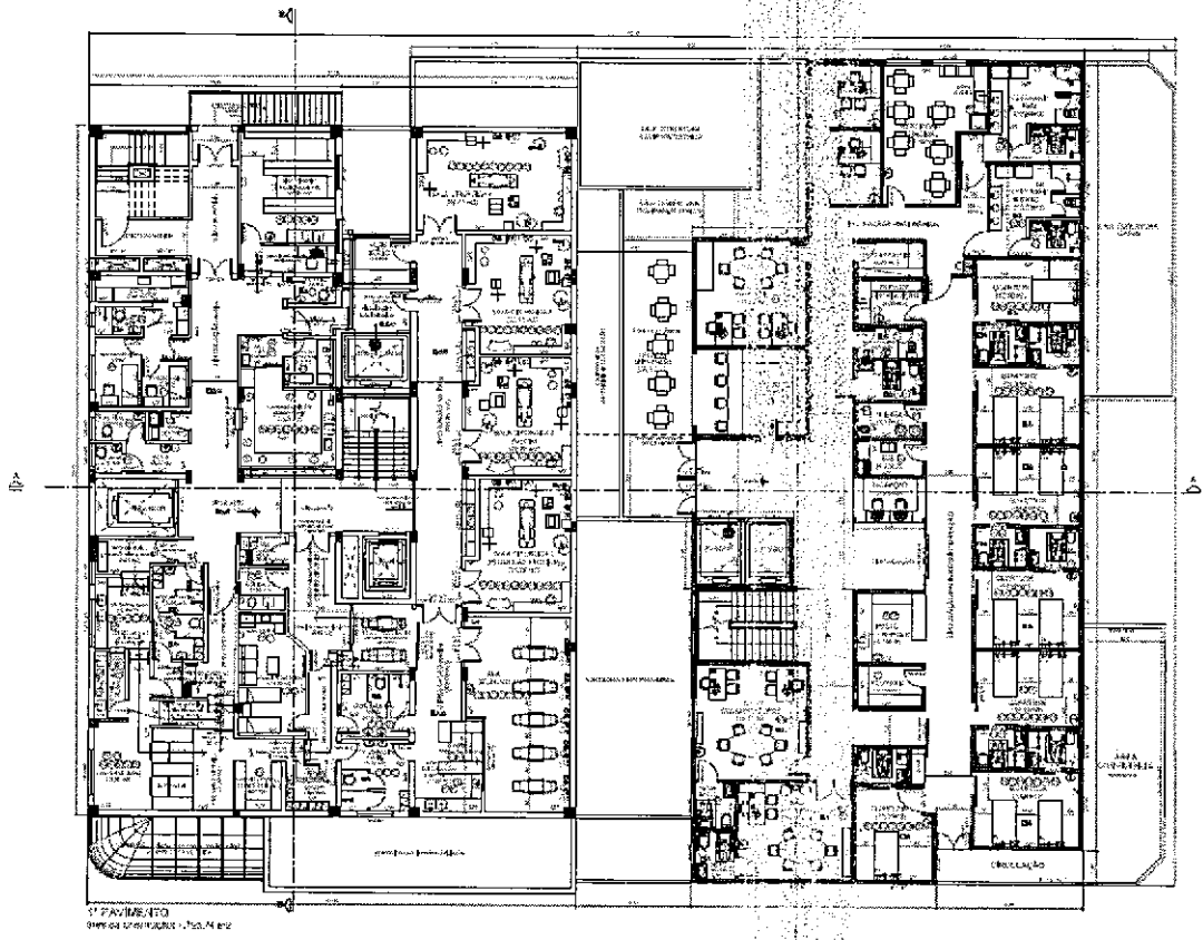
Figura 3: MEDCARE SUZANO SERVIÇOS MÉDICOS, croqui 1º PAVIMENTO
