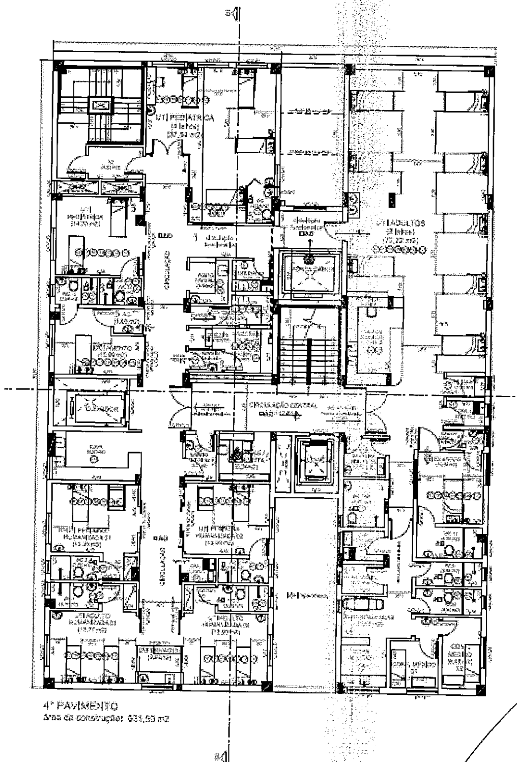
Figura 6: MEDCARE SUZANO SERVIÇOS MÉDICOS. croqui 4º PAVIMENTO
