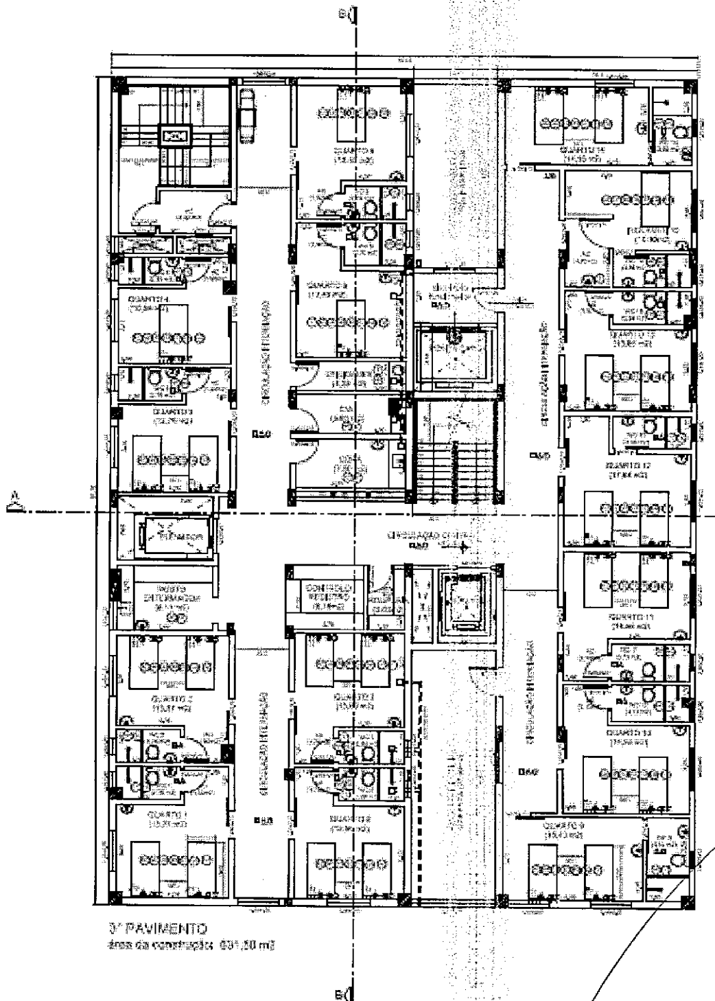
Figura 5: MEDCARE SUZANO SERVIÇOS MÉDICOS, croqui 3º PAVIMENTO
